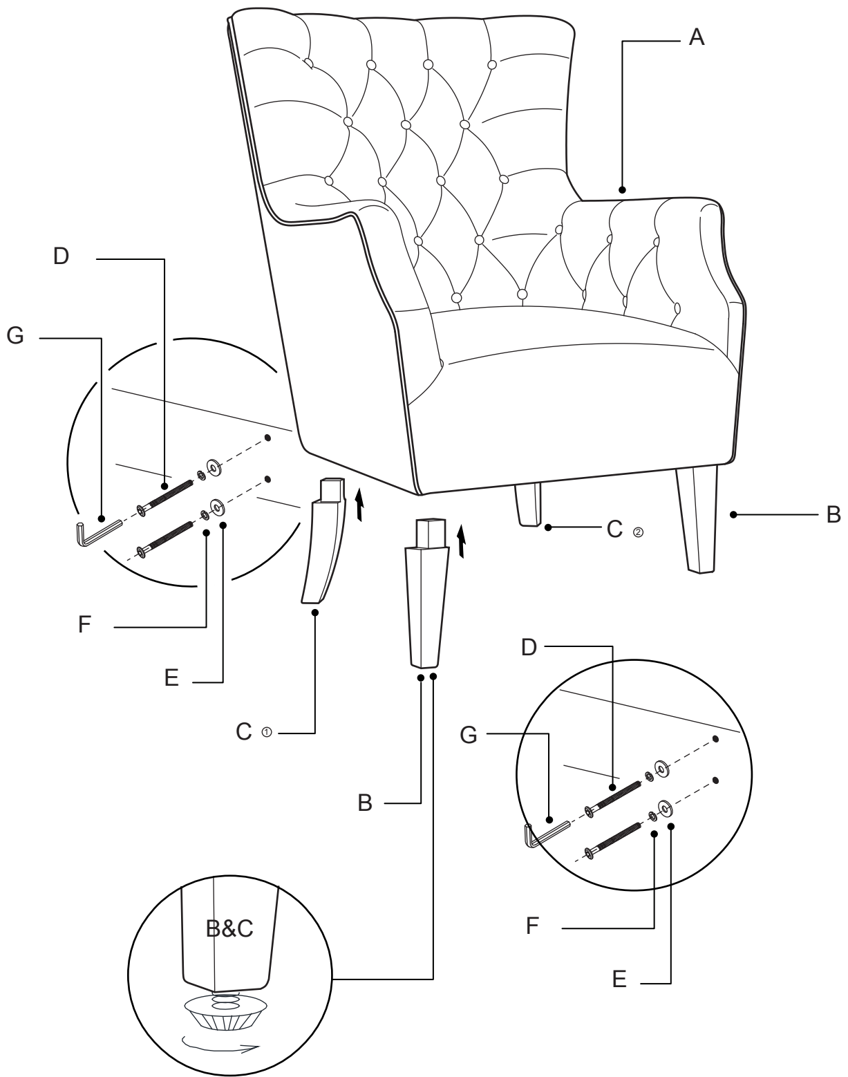
Adj.levelers
