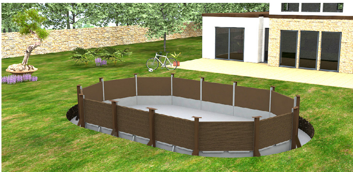
Mise en place de la traverse n° 2 jusqu'à la 6ème rangée.
